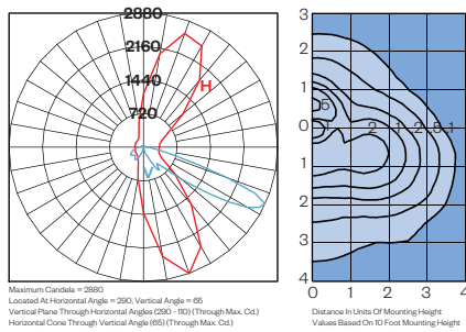
AO25PC-CL/AVI2-700MA-SO-27
