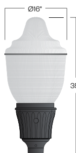
DUF1-ARP23
