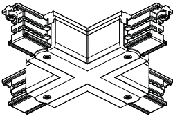
XTS38 - X Connector
