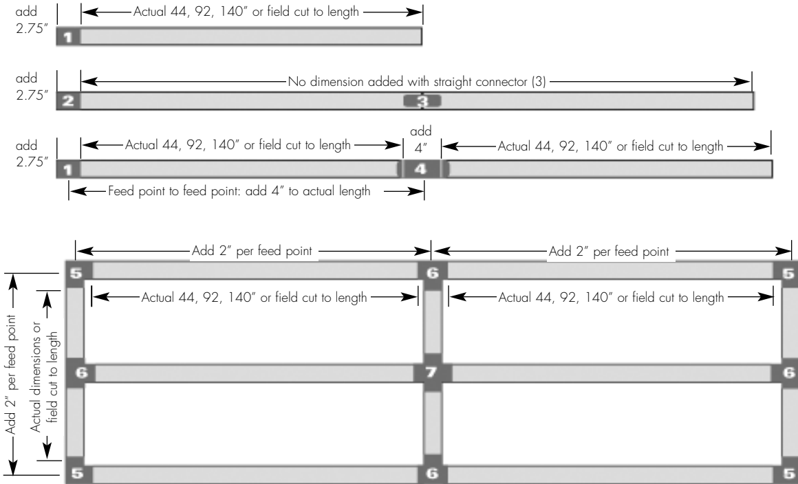
2. Conduit End Feed GES 13
